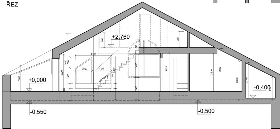
ŘEZ
